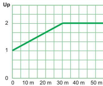
Fig. J54 : Tension maximale à l'extrémité d'un câble à vide en fonction de la longueur du câble pour un front de tension incident de 4kV/μs
