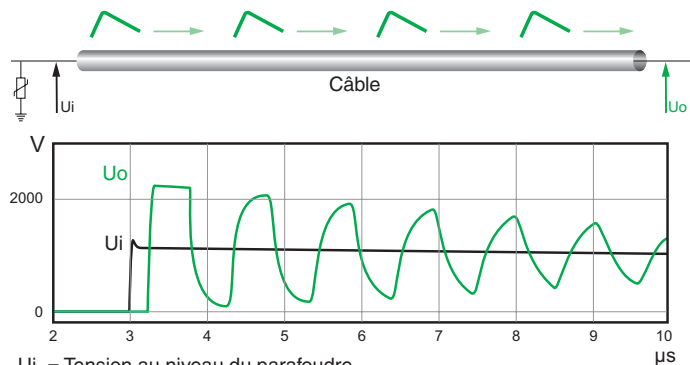
Fig. J53 : Réflexion d'une onde foudre à l'extrémité d'un câble
