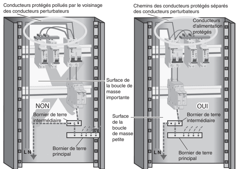
Fig. 42 : Exemple d'amélioration de la CEM par réduction des surfaces de boucle et de l'impédance commune au sein d'un coffret électrique
