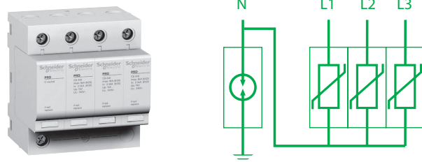
Fig. J47 : Le parafoudre PRD de marque Schneider Electric intègre un éclateur à gaz entre neutre et terre et des varistances entre phase et neutre
