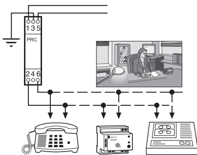
Fig. J44 : Réseau de télécommunication
