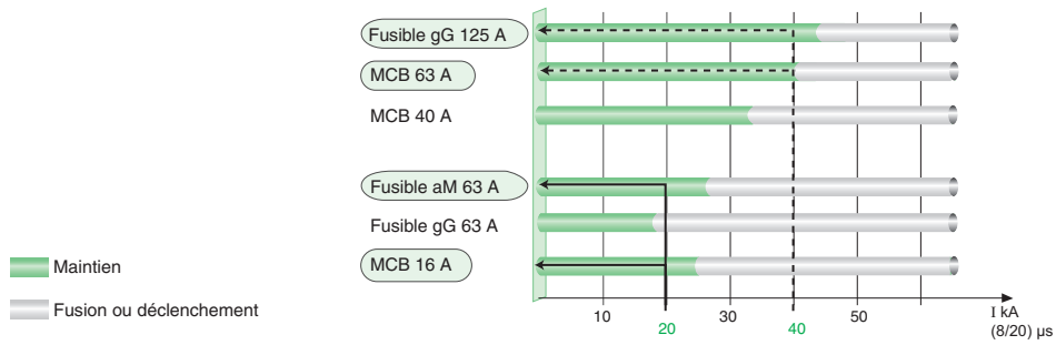
Fig. J50 : Comparaison des tenues à l'onde de tension pour un disjoncteur de 25 A et un fusible gG 63 A
