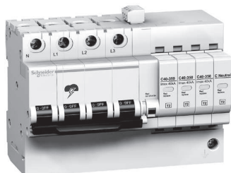
Fig. J48 : Parafoudre Quick PRD 3P +N de marque Schneider Electric
