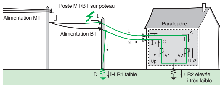
Fig. J55 : Protection seulement en mode commun
