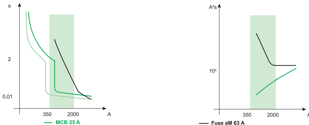
Fig. J51 : Comparaison des courbes temps/courant d'un disjoncteur et d'un fusible ayant les mêmes tenues à l'onde de courant 8/20 \mu s et comparaison des limitations en énergie d'un disjoncteur et d'un fusible ayant les mêmes tenues à l'onde de courant 8/20 \mu s
